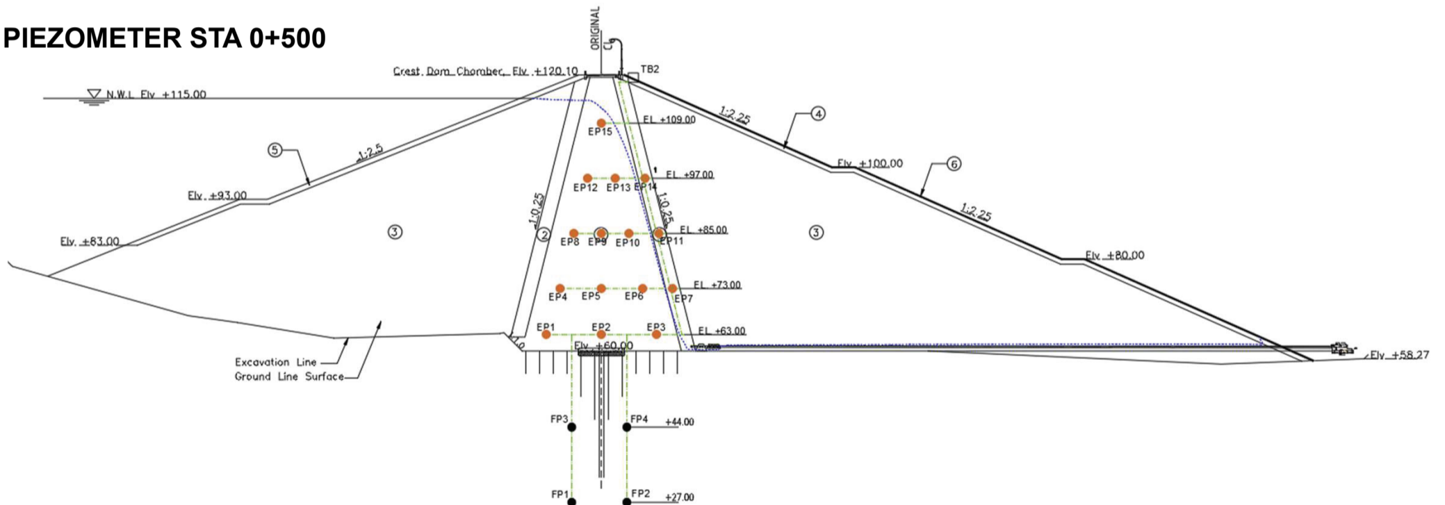
POTONGAN MELINTANG MAIN DAM EMBANKMENT PIEZOMETER (EP) DAN FOUNDATION PIEZOMETER (FP) STA. 0+500
